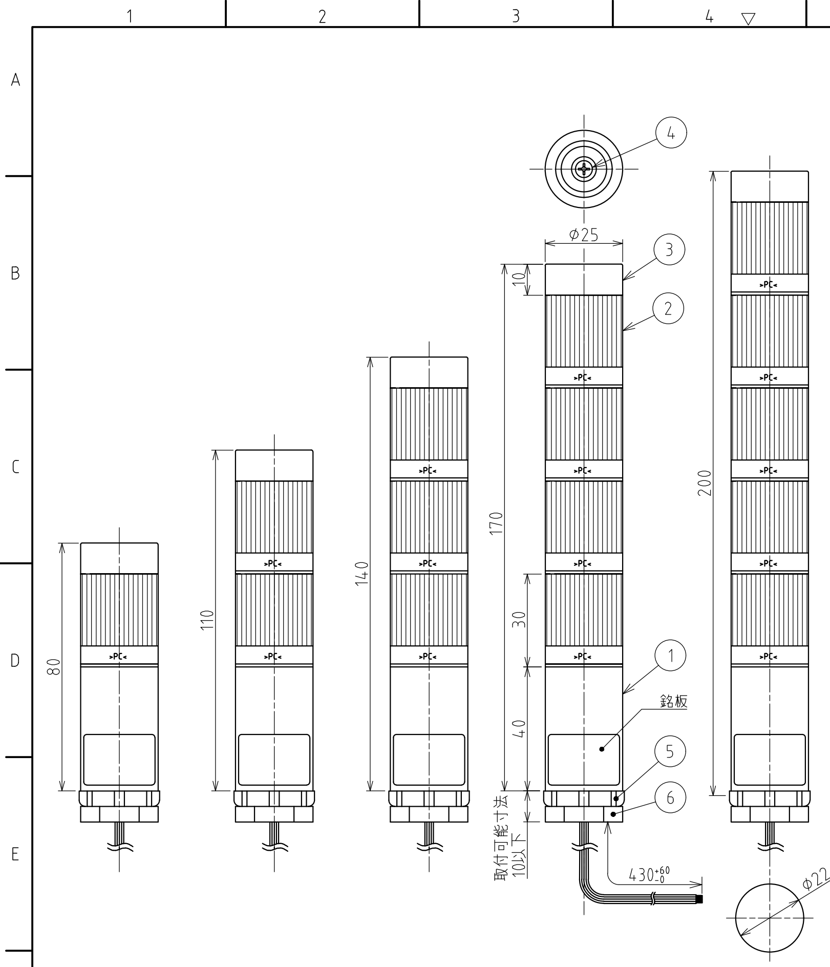
取付面寸法図
